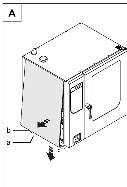
Bild: Seitenwand abnehmen: A: Größe 6.x und 10.x, B: Größe 20.x
