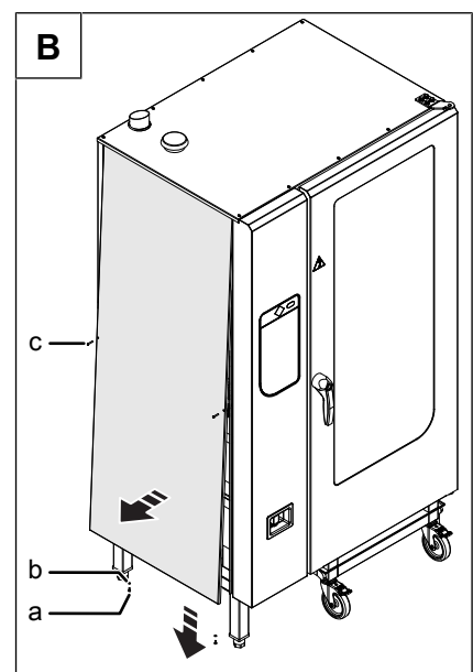
Bild: Seitenwand abnehmen: A: Größe 6.x und 10.x, B: Größe 20.x
