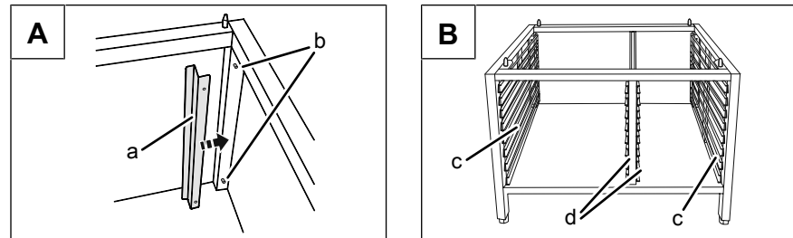
Bild: A Anschlagprofil, B Eihängegestell
